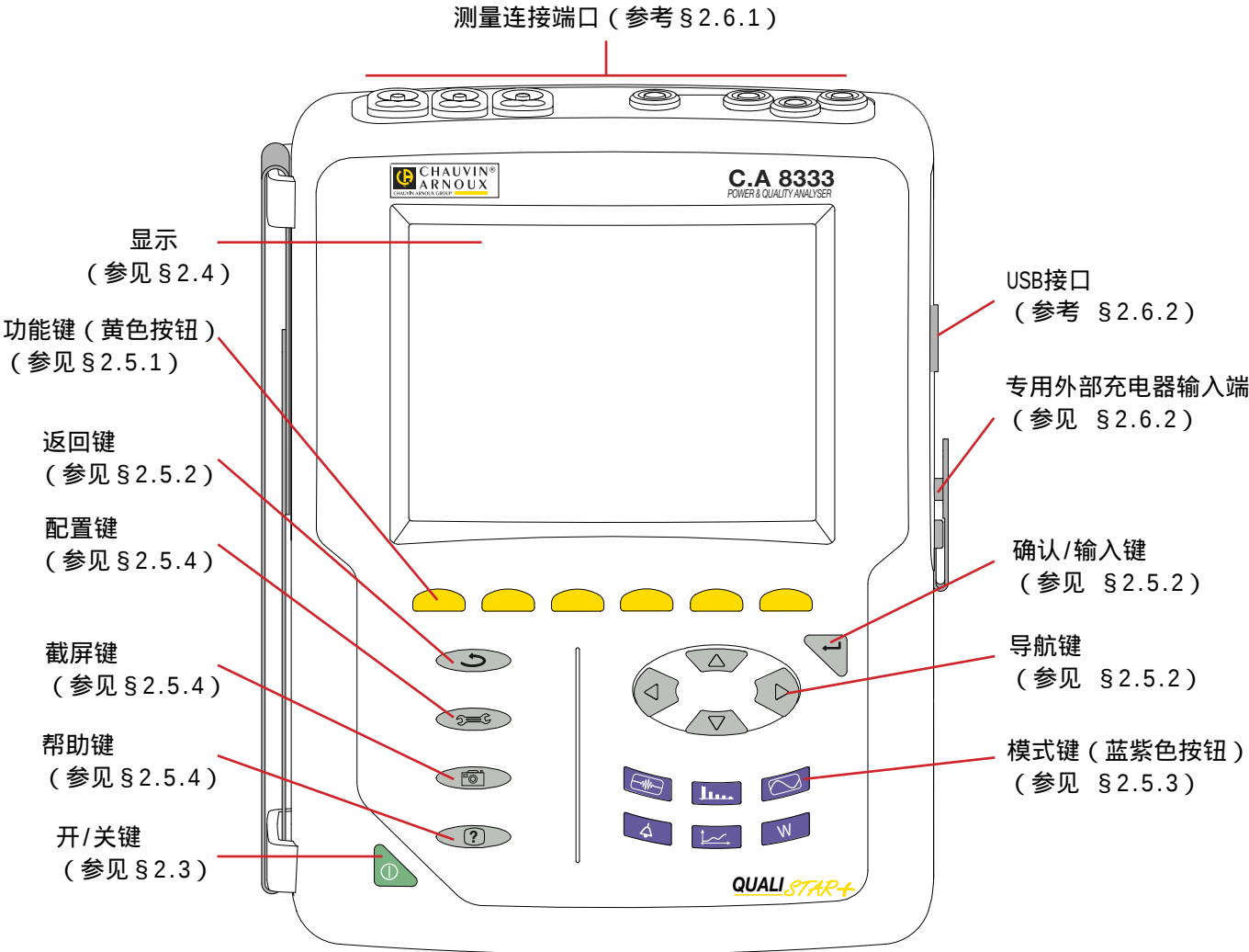
图2：仪器全览
