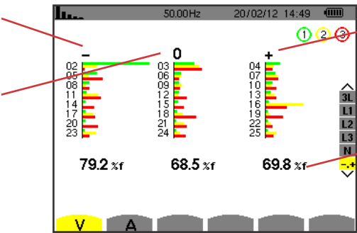
图50: 相电压专家模式页面 (含中性线三相结构)
