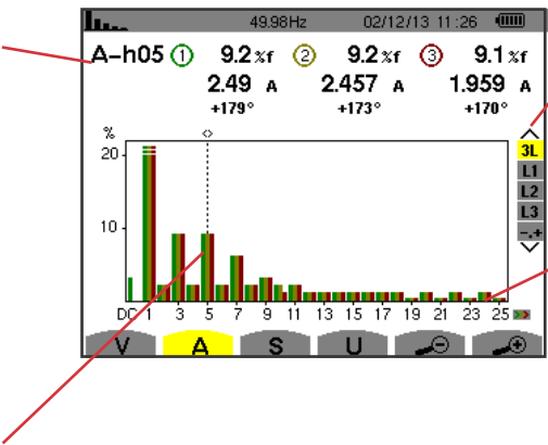
图 44: 3L 电流谐波显示举例
