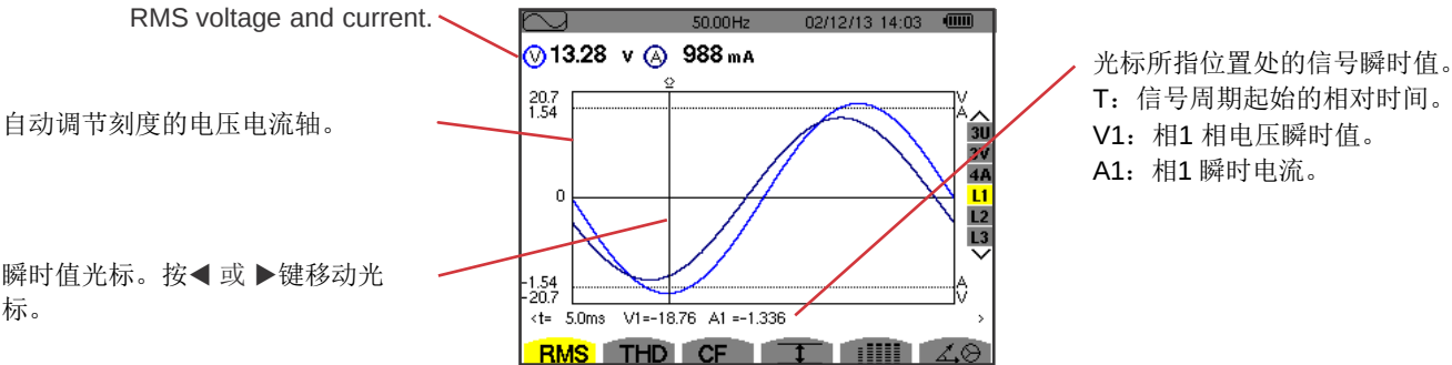
图56: L1 RMS显示页面
